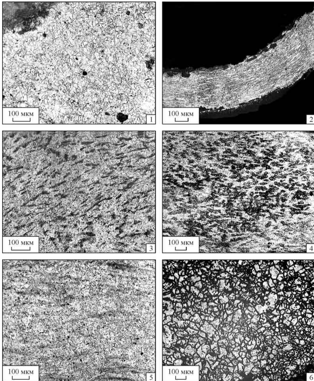
Рис. 3.5. Мікроструктури: 1 — ан. 290; 2 — ан. 289а; 3 — ан. 289б; 4 — ан. 295; 5 — ан. 299; 6 — ан. 297
